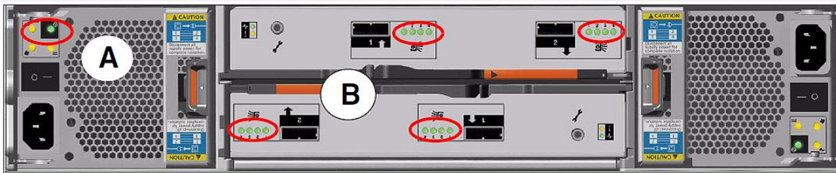
Storwize v7000 expansion enclosure: вид сзади
